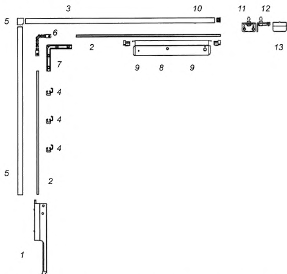
1 — ручка; 2 — соединительная тяга, 3 — декоративная накладка тяги; 4 — направляющая откидная тяга; 5 — угловая накладка; 6 — угловая цепная передача; 7 — направляющая угловой передачи; 8 — ножницы, 9 — торцевые заглушки ножниц; 10 — торцевая заглушка накладки; 11 — высокий створчатый кронштейн для поливинилхлоридных и алюминиевых профилей, 12 — плоский створчатый кронштейн для деревянных профилей; 13 — накладка кронштейна
