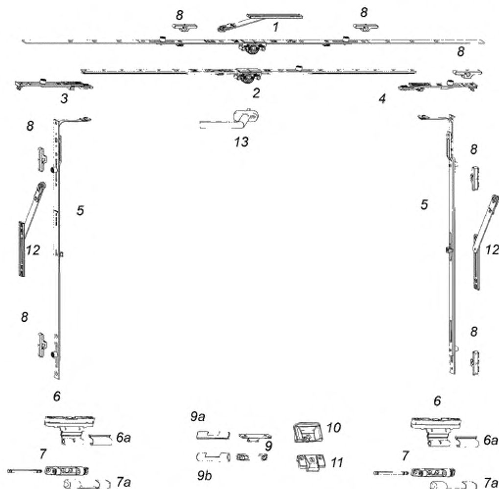
1 — основной поворотный средний запор; 2 — основной поворотно-откидной средний запор; 3 — шпингалет основного запора; 4 — шпингалет основного запора 90°; 5 — средний запор; 6 — средняя регулируемая петля на створке; 6a — декоративная накладка верхней петли на створке; 7 — верхняя петля на раме со штифтом; 7a — декоративная накладка верхней петли на раме; 8 — ответная планка; 9 — средний накладной прижим; 9a — декоративная створочная накладка среднего прижима; 9b — декоративная рамная накладка среднего прижима; 10 — средний скрытый прижим, створочная часть; 11 — средний скрытый прижим, рамная часть; 12 — фрамужные ножницы; 13 — ручка
