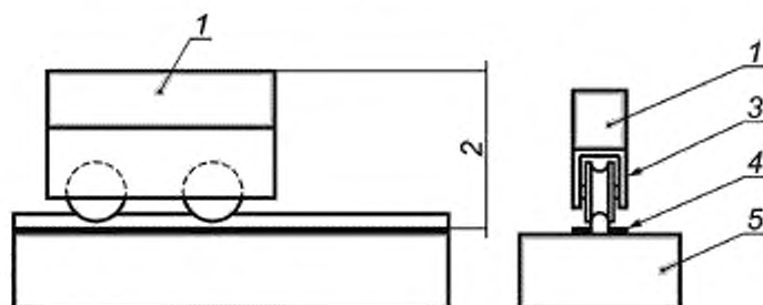
Рисунок Е.1 — Схема испытания роликов на надежность
