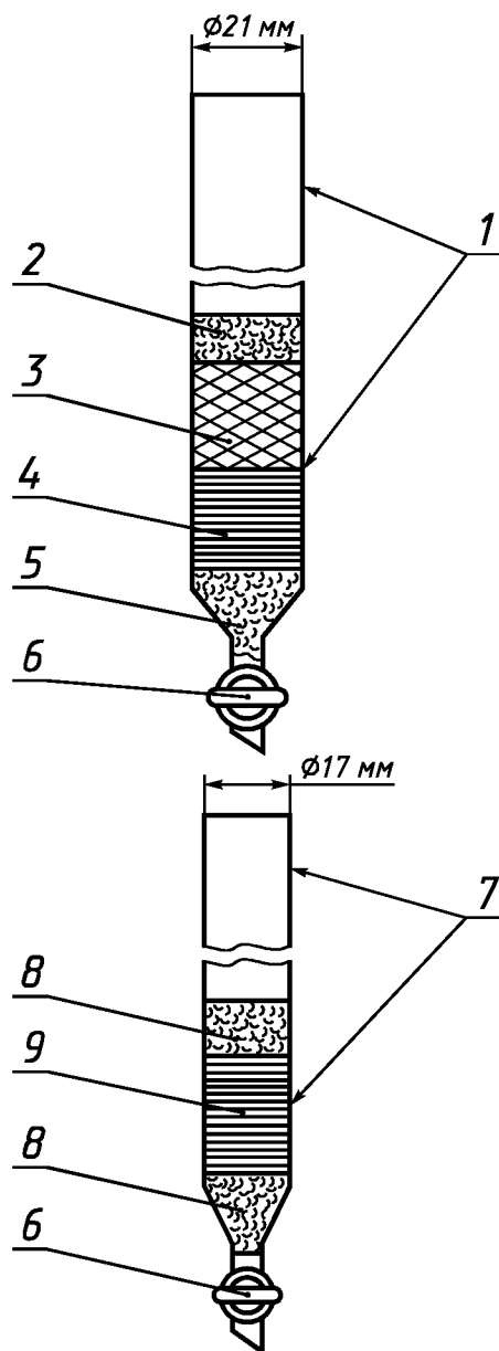
1 — колонка 1 (щелочная), длина 250 мм; 2 — хлопковая вата или стекловата; 3 — смесь диатомовой земли и анализируемого образца; 4 — 3 г диатомовой земли и 2 см 3 NaOH (5,16 г); 5 — хлопковая вата или стекловата; 6 — кран, предпочтительно из политетрафторэтилена; 7 — колонка 2 (кислотная), длина 250 мм; 8 — стекловата; 9 — 3 г диатомовой земли и 3 см 3 H 2 SO 4 (6,36 г)
