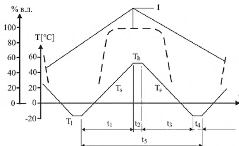
1 — относительная влажность в течение температурного цикла; T_h — температура выдержки, равная (53,0 \pm 2,0)^\circ\text{C} ; T_l — температура выдержки, равная минус (18,0 \pm 2,0)^\circ\text{C} ; T_s — перепад температур, равный (14 \pm 2,0)^\circ\text{C} в течение часа; t — интервалы времени
