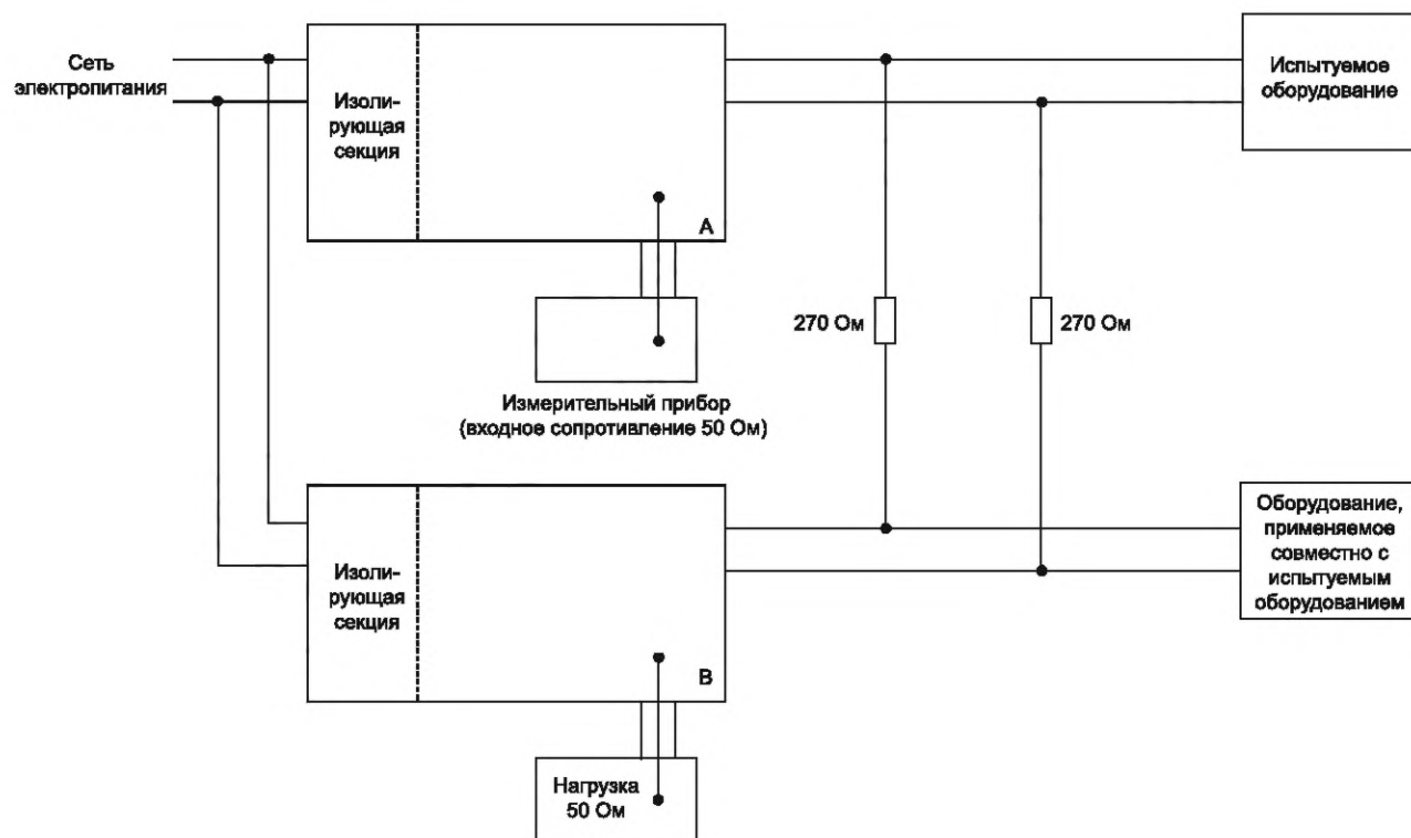
А, В — эквиваленты сети по ГОСТ 30847 (типы 1, 4)
