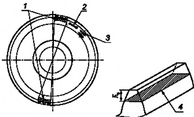
1 — поперечный темплет, 2 — один образец на растяжение ГОСТ 1497, тип III; 3 — два образца на ударную вязкость при t = +20 °C ГОСТ 9454, тип 1; 4 — продольный темплет
