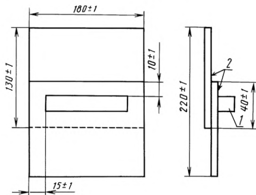
1 — электрод; 2 — лицевая сторона тентового материала
