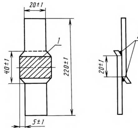
1 — сварной шов; 2 — выпрессовка
