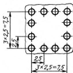
Установочные размеры
