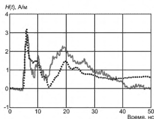
Рисунок D.7 — Сравнение значений напряженности магнитного поля, вычисленных по результатам измерений напряжения в петлевом сенсоре (сплошная линия) и методом чисового моделирования (пунктирная линия) (электростатический разряд на расстоянии 45 см от сенсора)
