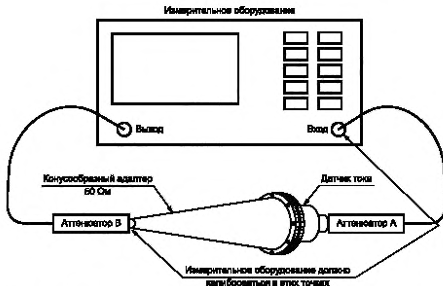
Рисунок В.3 — Схема измерения вносимого затухания цепи «датчик тока — аттенуатор — кабель»
