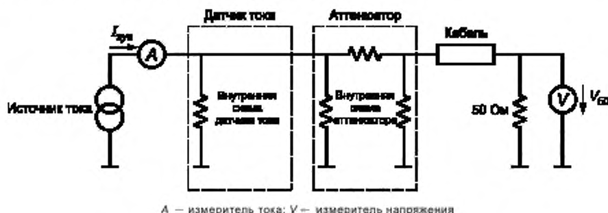
Рисунок В.4 — Схема определения низкочастотного передаточного сопротивления системы измерения тока
