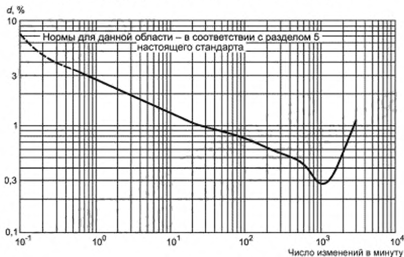
Рисунок 3 — Характеристика относительного изменения напряжения
