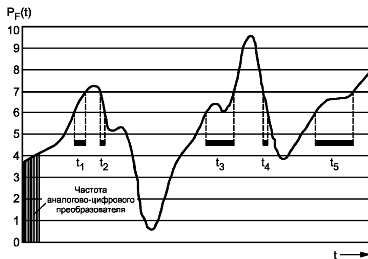
Рисунок 2а — Уровень фликера как функция времени
