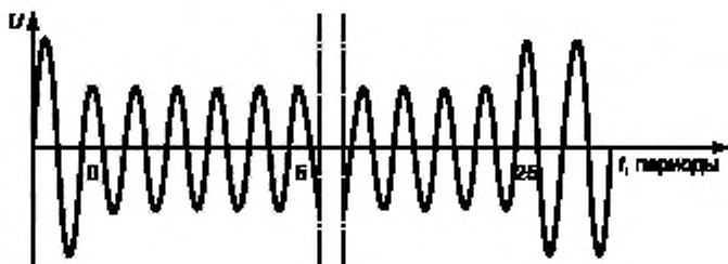
а) Форма провала напряжения при понижении напряжения до 70 % U_T в течение 25 периодов при переходе через нуль
