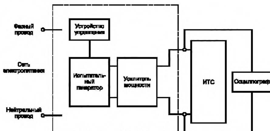
в) Схема испытаний с использованием усилителя мощности
