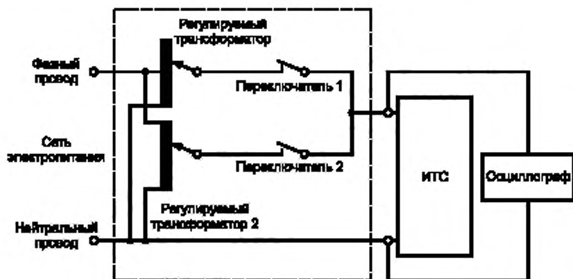
а) Схема испытаний с использованием регулируемых трансформаторов и переключателей
