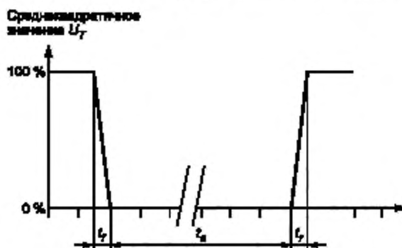
Рисунок 2 — Кратковременное прерывание напряжения
