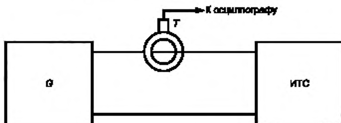
Рисунок А.1 — Схема измерения пикового значения нагрузочного тока ИГ кратковременных прерываний напряжения
