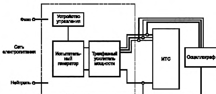
Рисунок С.2 — Схема установки для испытаний трехфазных систем при воздействии провалов, кратковременных прерываний и изменений напряжения электропитания
