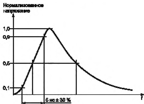
Рисунок 3 — Форма импульсов напряжения на выходе ИГ при нагрузке 50 Ом
