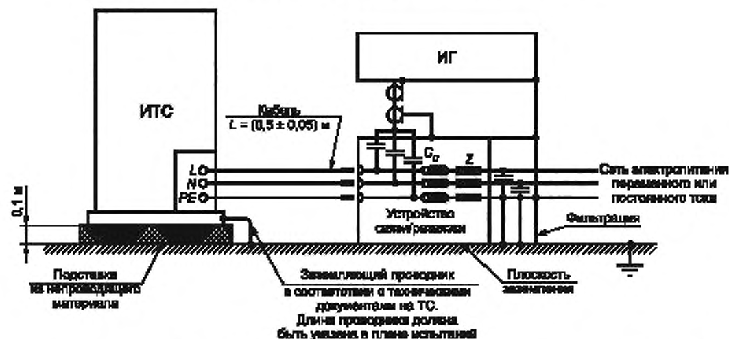
Рисунок 8 — Пример установки для испытания оборудования в стойке
