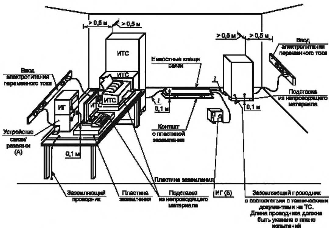
Рисунок 6 — Схема испытаний ТС на устойчивость к НИП
