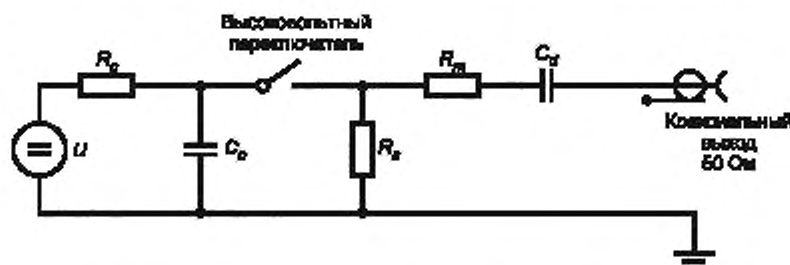
Рисунок 1 — Упрощенная схема ИГ
