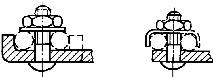
г. Зажим с прижимной планкой
