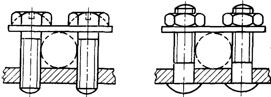
г. Зажим с прижимной планкой
