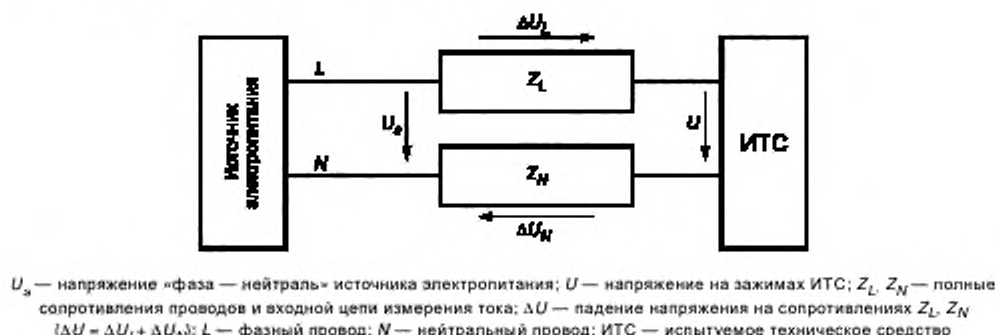
Рисунок 2 — Схема измерений эмиссии в однофазных системах
