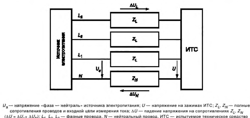
Рисунок 3 — Схема измерений эмиссии в трехфазных системах
