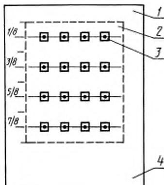
Расположение медных пластин
