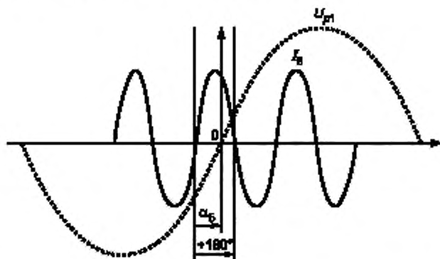
Рисунок 1 — Определение угла фазового сдвига гармонической составляющей тока 5-го порядка I_5 относительно основной составляющей фазного напряжения U_{p1} ( I_5 опережает U_{p1} , \alpha_5 > 0 )
