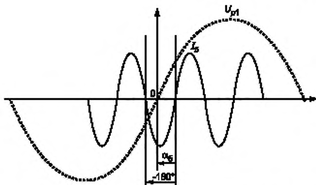
Рисунок 2 — Определение угла фазового сдвига гармонической составляющей тока 5-го порядка I_5 относительно основной составляющей фазного напряжения U_{p1} ( I_5 отстает от U_{p1} , \alpha_5 < 0 )
