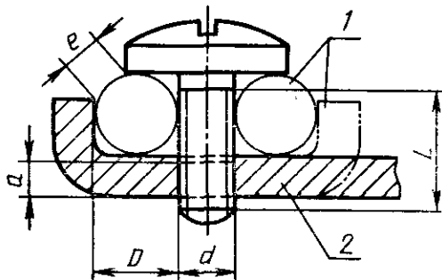
Винт, не требующий шайбы или прижимной пластины
