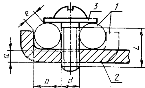
Винт, требующий шайбу или прижимную пластину
