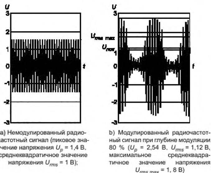
Рисунок 1 — Определение степени жесткости испытаний и формы колебаний на выходе генератора сигналов
