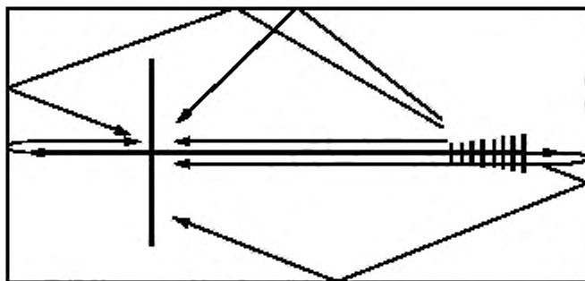
Рисунок С.1 — Многочисленные отражения в существующих малых безэховых камерах
