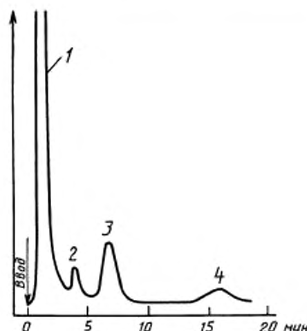
Типовая хроматограмма этиленгликоля с использованием колонки I
