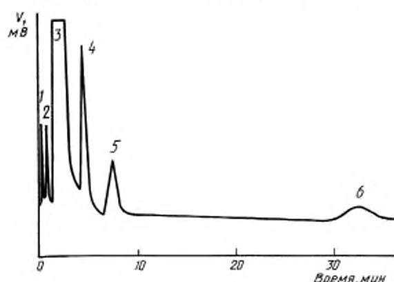
Типовая хроматограмма этиленгликоля с использованием колонки II
