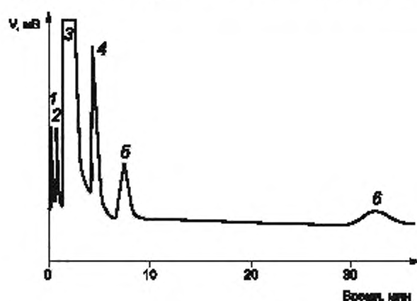
1, 2 — неидентифицированные примеси; 3 — этиленгликоль; 4 — бензиловый спирт (внутренний эталон); 5 — диэтиленгликоль; 6 — триэтиленгликоль
