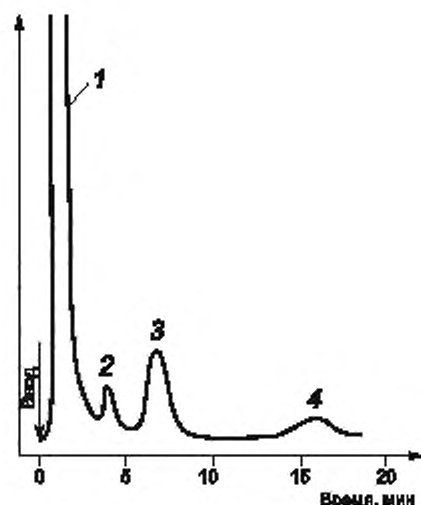
1 — этиленгликоль; 2 — диэтиленгликоль; 3 — нонанол-1 (внутренний эталон); 4 — триэтиленгликоль
