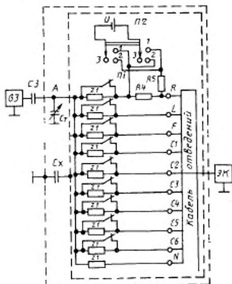
Схема определения коэффициента ослабления синфазных сигналов
