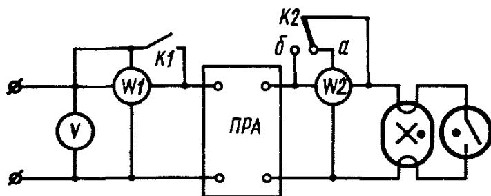
V —вольтметр, измеряющий напряжение сети; W1 —ваттметр, измеряющий мощность потребляемую из сети; W2 —ваттметр, измеряющий мощность лампы; K1 —ключ однополюсный; K2 —переключатель.
