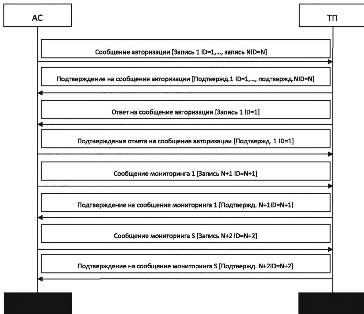
Рисунок 7 — Диаграмма обмена сообщениями
