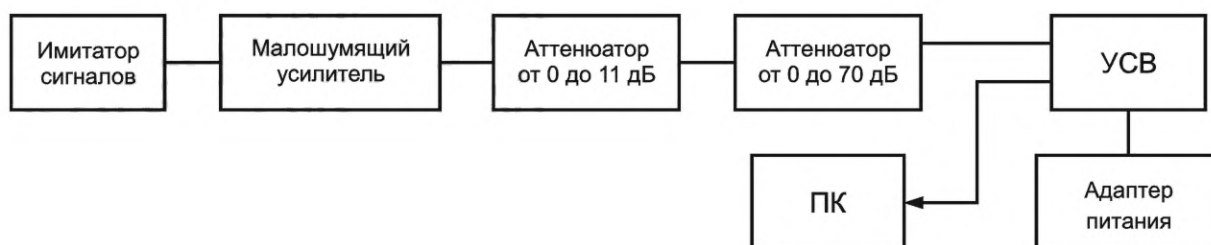
Рисунок В.3 — Схема определения чувствительности модуля ГНСС
