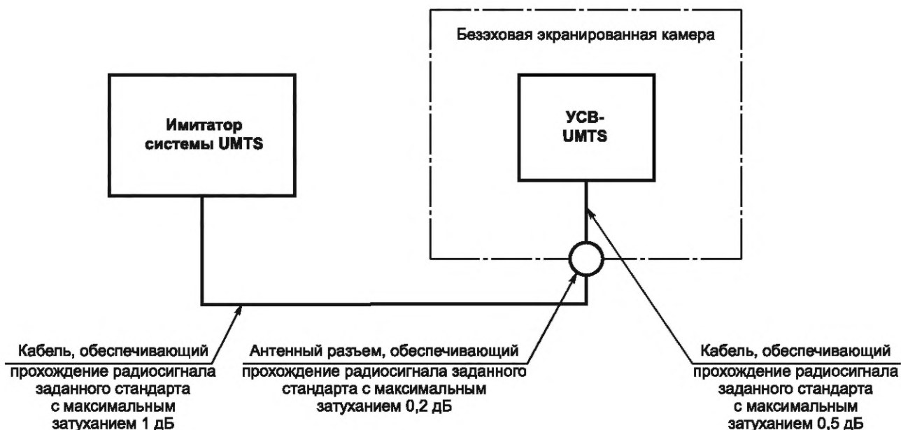
Рисунок Д.1 — Схема испытаний UCSB-UMTS с использованием имитатора системы UMTS
