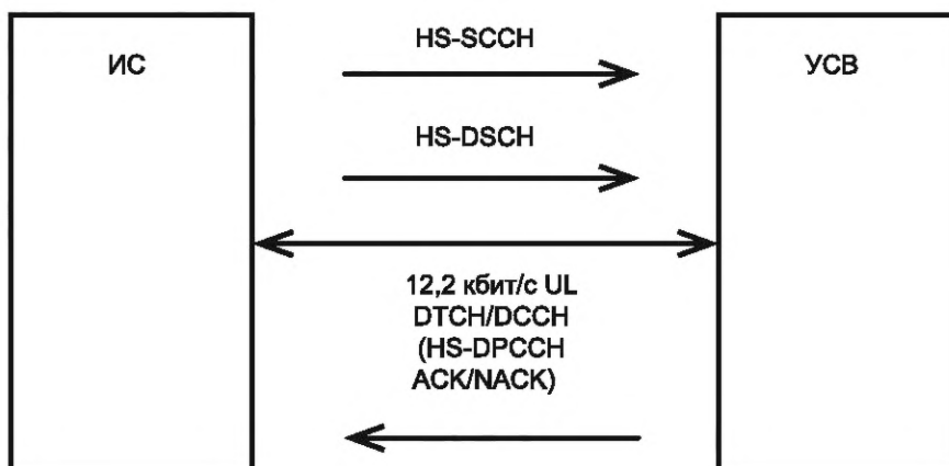
Рисунок Д.2 — Схема испытаний UCSB-UMTS для определения предельно допустимой максимальной мощности в режиме HSDPA
