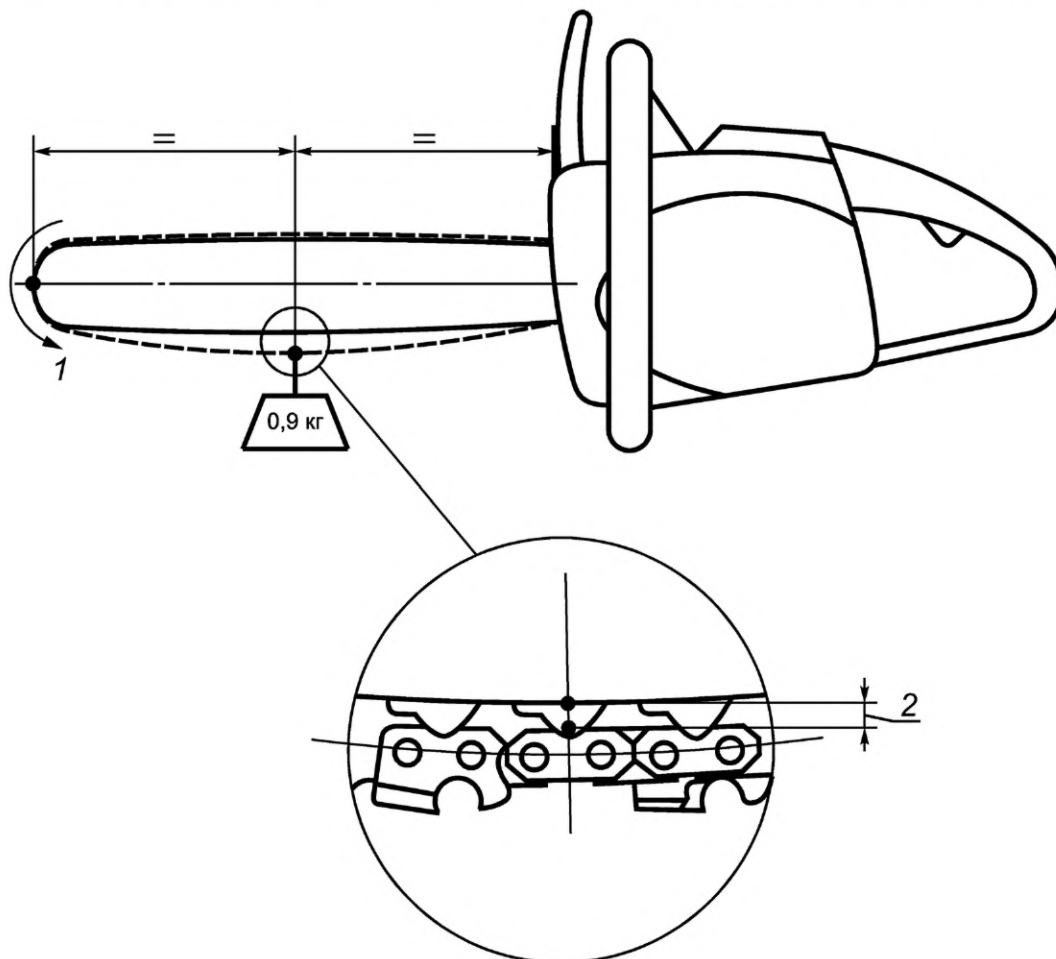
Рисунок 3 — Регулировка натяжения цепи
