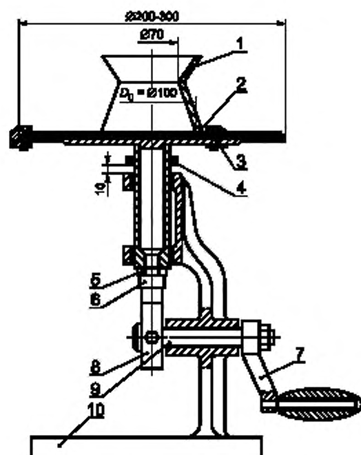
1 — форма-конус с воронкой; 2 — стекло; 3 — стол; 4 — упорное кольцо; 5 — стопорная гайка; 6 — упор; 7 — ручка; 8 — кулачок (эксцентрик); 9 — валик; 10 — станина с приводом
