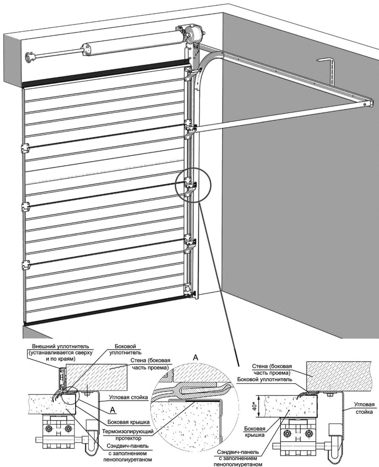
Рисунок Д.3 — Сечение секционных ворот (3D)
