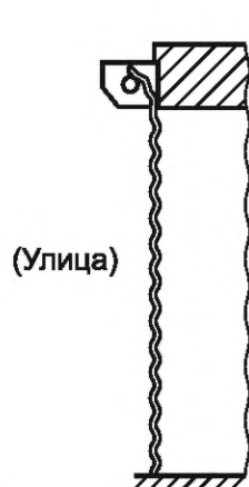
Полотно вне проема, устройство намотки с защитным коробом снаружи
