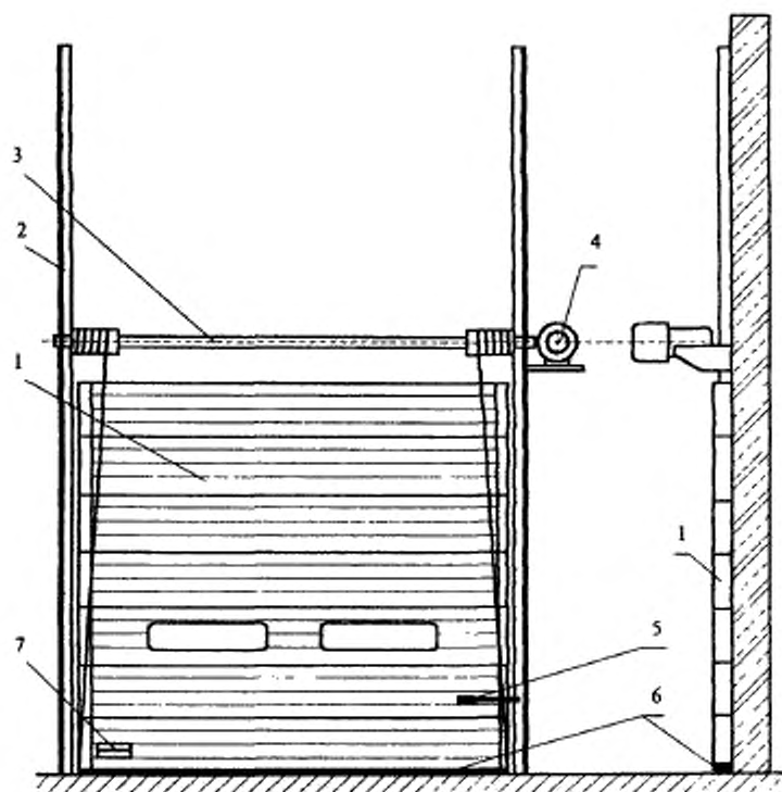
1 — полотно ворот; 2 — направляющие профили; 3 — система уравнивания полотна; 4 — привод; 5 — задвижка; 6 — уплотнители; 7 — ручка
