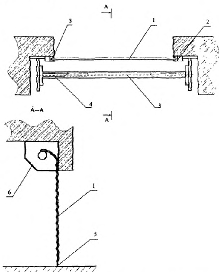
Рисунок А.8 — Пример конструкции рулонных роллетных ворот
