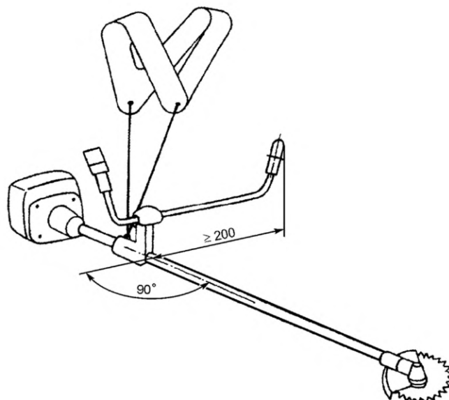
Рисунок 4 — Кусторе́з, ручка которого служит защитным устройством
