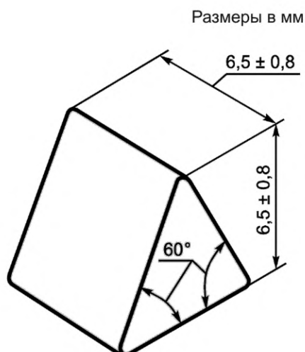
Рисунок Б.3 — Предмет испытания
