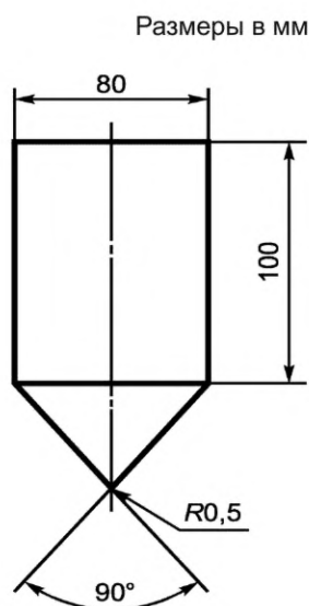
Рисунок 6 — Испытательный конус
