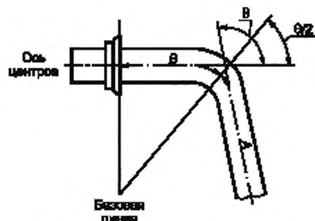
Рисунок 1 — Основные параметры трахеотомической трубки
