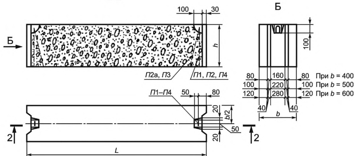
Рисунок 1 — Блоки типа ФБС
