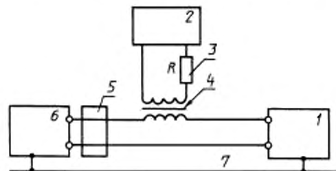
I — испытуемое изделие; 2 — генератор; 3 — сопротивление связи, R = 40 Ом; 4 — соединительный трансформатор; 5 — дополнительное средство защиты от помех; 6 — внешнее устройство; 7 — опорная земля
