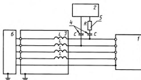
I — испытуемое изделие; 2 — генератор; 3 — разделительное устройство, L = 1,5 мГн; 4 — конденсаторы связи, C = 0,5 мкФ (2 шт.); 5 — сопротивление связи, R = 40 Ом; 6 — внешнее устройство
