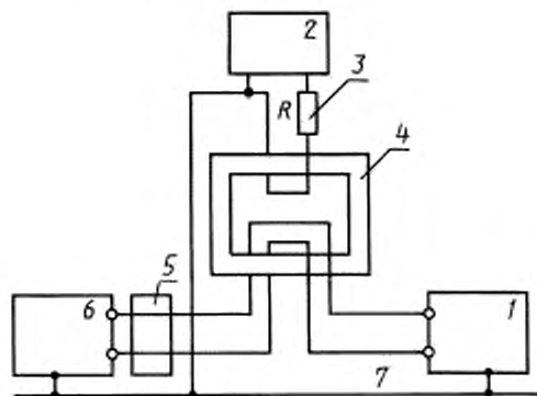
I — испытуемое изделие; 2 — генератор; 3 — сопротивление связи, R = 40 Ом; 4 — индуктивное устройство; 5 — дополнительное средство защиты от помех; 6 — внешнее устройство; 7 — опорная земля
