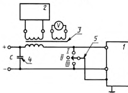
1 — испытуемое изделие; 2 — генератор; 3 — соединительный трансформатор; 4 — конденсатор, C = 47 \text{ мкФ} ; 5 — переключатель (I и II — несимметричная помеха; III — симметричная помеха)
