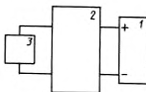
1 — испытуемое изделие; 2 — имитатор помех; 3 — блок питания
