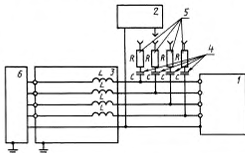
I — испытуемое изделие; 2 — генератор; 3 — разделительное устройство, L = 1,5 мГн; 4 — конденсаторы связи, C = 0,5 мкФ (4 шт.); 5 — сопротивление связи, R = 40 Ом (4 шт.); 6 — внешнее устройство
