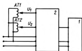
1 — испытуемое изделие; 2 — имитатор помех; AT1, AT2 — автотрансформаторы
