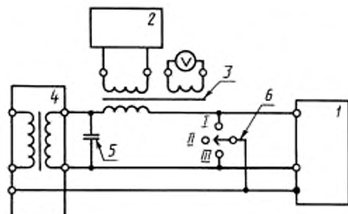
1 — испытуемое изделие; 2 — генератор; 3 — соединительный трансформатор; 4 — разделительный трансформатор; 5 — конденсатор, C = 47 \text{ мкФ} ; 6 — переключатель (I — фаза—земля, II — фаза—фаза, III — нейтраль—земля)
