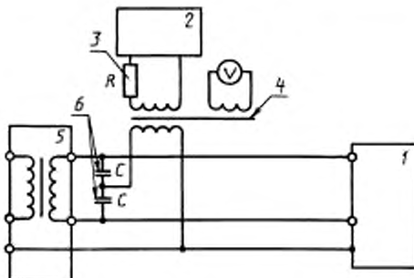
1 — испытуемое изделие; 2 — генератор; 3 — соединительный трансформатор; 4 — разделительный трансформатор; 5 — конденсатор, C = 47 \text{ мкФ} ; 6 — переключатель (I — фаза—земля, II — фаза—фаза, III — нейтраль—земля)
