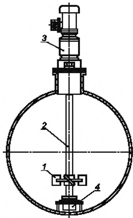
1 — мешалка; 2 — вал; 3 — мотор-редуктор; 4 — подпятник
