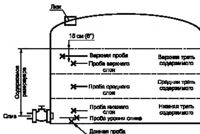
Рисунок 11 — Отбор проб из больших емкостей
