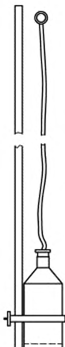
Рисунок 6 — Бутылка для отбора проб
