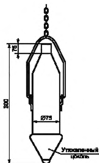
Рисунок 10 — Утяжеленная бутылка для отбора проб
