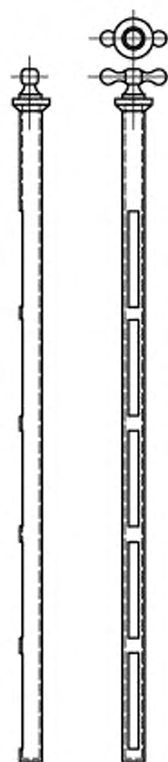
Рисунок 3 — Пробоотборник, состоящий из двух концентрических трубок
