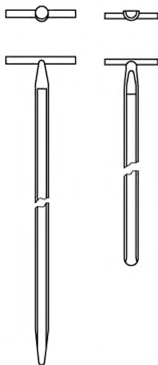
Рисунок 2 — Совковые пробоотборники для взятия проб порошков
