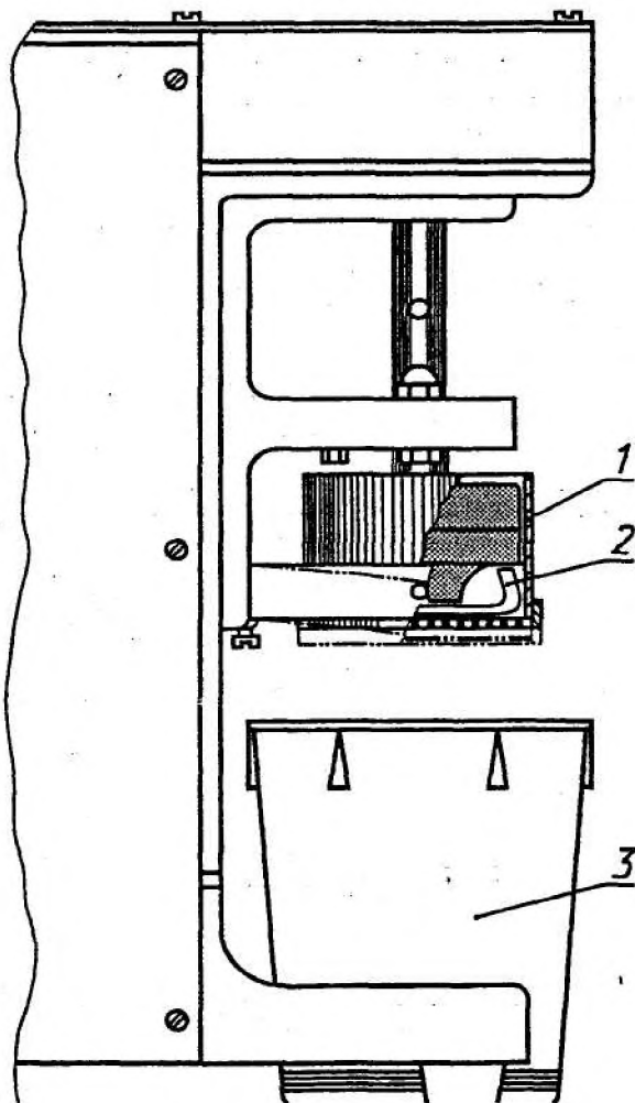
Рисунок 1 — Автоматический прибор для отделения клейковины
