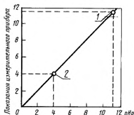
1 — показание измерительного прибора с щелочным безводным буфером равно 11,5; 2 — измерительный прибор, отрегулированный на показание 4,0 в кислотном безводном буфере
