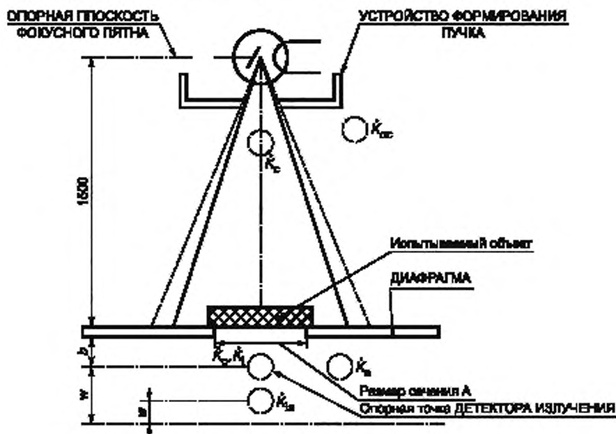
Рисунок 1 — Геометрия ШИРОКОГО пучка.
