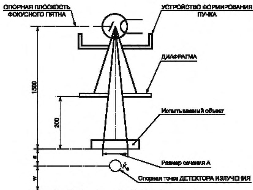
Рисунок 2 — Геометрия УЗКОГО ПУЧКА
