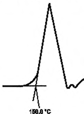
Точку плавления (156,6 °С) определяют в точке пересечения продолжения линии начала пика и продолжения базовой линии
