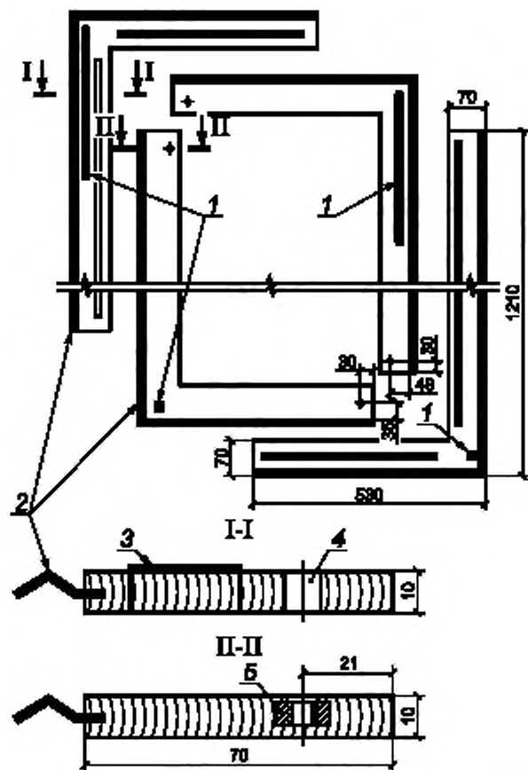
Рисунок 1 — Элементы раздвижной деревянной рамы
