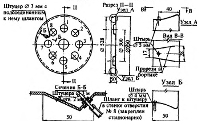
Рисунок 4 — Пластина с отверстиями к кожуху вентилятора
