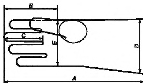
Рисунок 1 — Внутренние размеры ЗАЩИТНЫХ ПЕРЧАТОК
