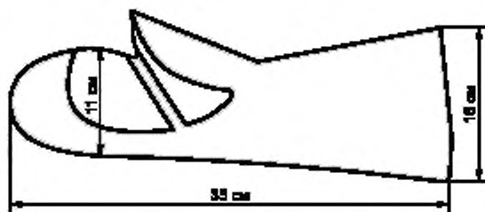
Рисунок 2 — Внутренние минимальные размеры ЗАЩИТНЫХ РУКАВИЦ
