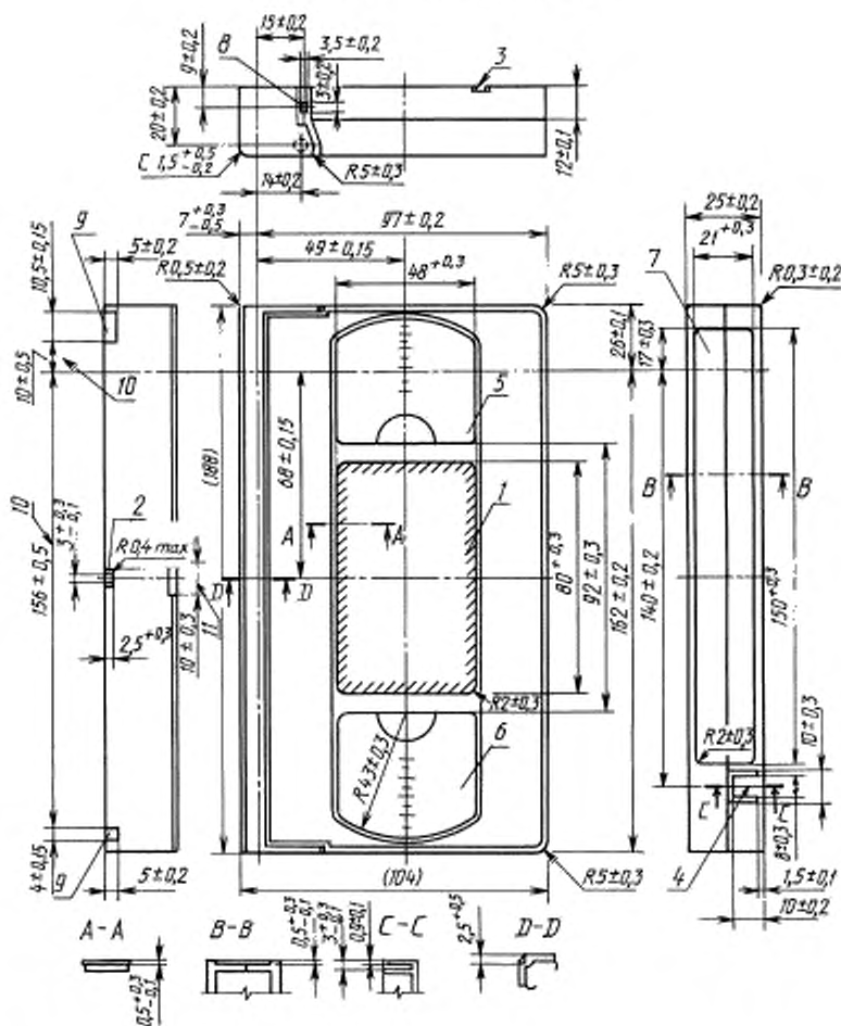
Видеокассета. Вид сверху и сбоку
