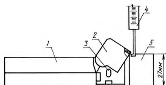
1 — видеокассета; 2 — защитная крышка; 3 — защелка; 4 — динамометр; 5 — ограничительный калибр
