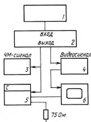
Схема измерений
