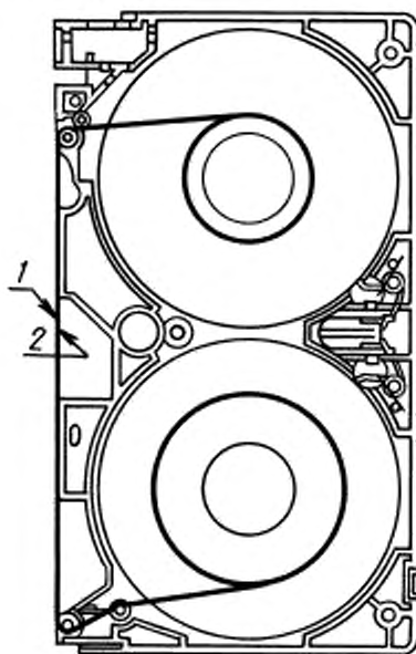
Траектория движения магнитной ленты
