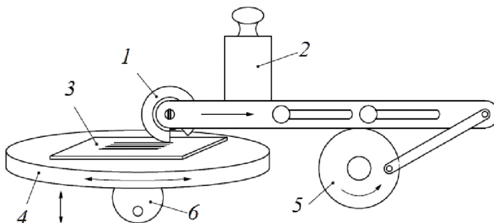
1 – режущий инструмент; 2 – груз; 3 – испытываемая пластинка; 4 – вращающаяся подставка для испытываемой пластинки; 5 – мотор; 6 – ручка для вращения подставки
