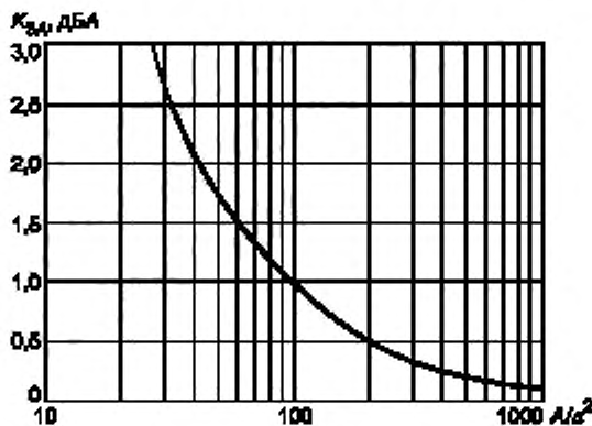
Рисунок А.1 — Локальная коррекция на акустические условия K_{3,4} в зависимости от A/a^2
