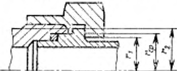
в) Фланцевое соединение
