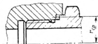
в) Фланцевое соединение
