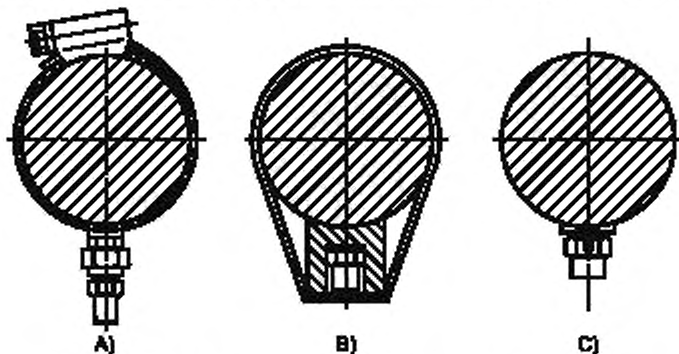
Рисунок 2 — Способы крепления датчика вибрации
