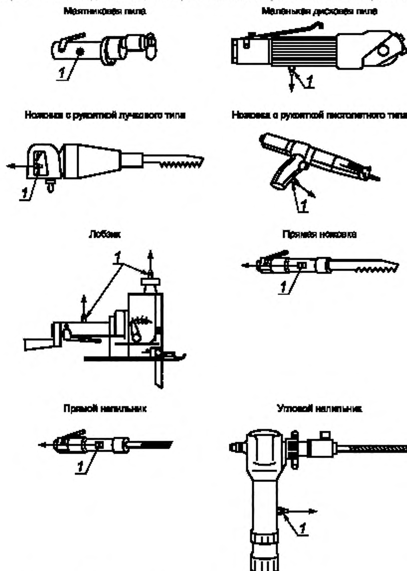
Рисунок 2 — Направления измерений и примеры размещения датчиков вибрации
