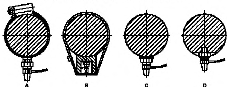
Рисунок 1 — Способы крепления датчика вибрации
