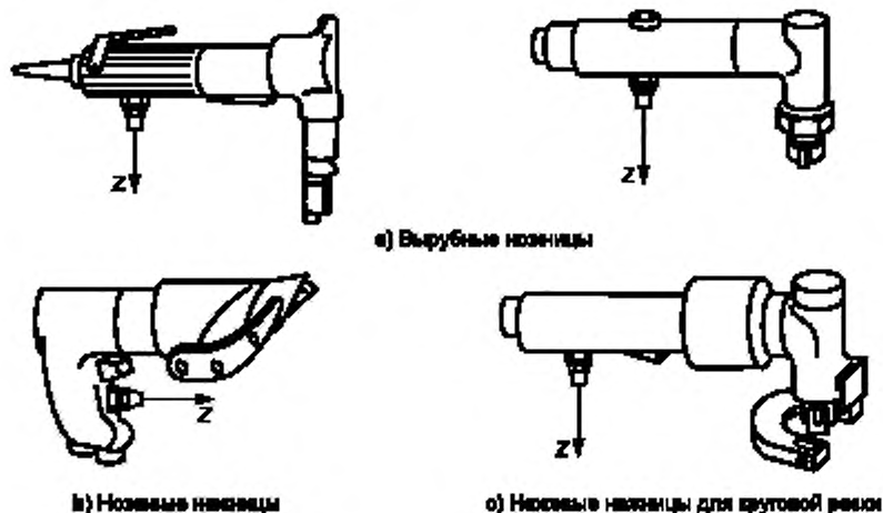
Рисунок 2 — Направления измерений и примеры размещения датчика вибрации
