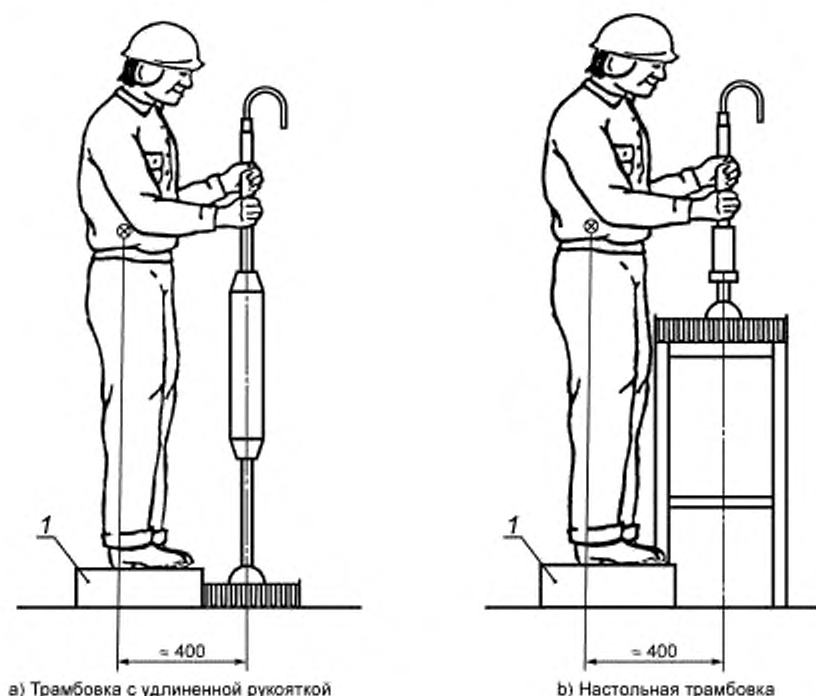
Рисунок 3 — Рабочая поза оператора
