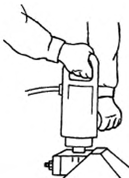
е) Ручная машина с основной и поддерживающей рукоятками [см. рисунки 3б), в центре и справа, и 3с), в центре и справа] (рука оператора на поддерживающей рукоятке, насколько возможно, параллельна оси двигателя)
