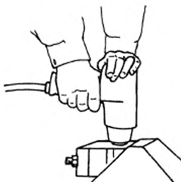
д) Ручная машина с рукояткой пистолетного или лучкового типа, без поддерживающей рукоятки [см. рисунки 3б), слева и 3с), слева] и хвостовиком размером свыше 10 мм (оператор выполняет задание с использованием обеих рук)
