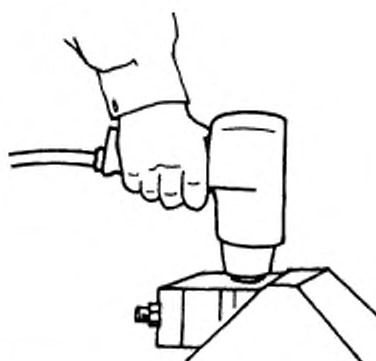
в) Ручная машина с рукояткой пистолетного типа, без поддерживающей рукоятки [см. рисунок 3б), слева] и хвостовиком размером до 10 мм включительно (оператор удерживает ручную машину одной рукой)
